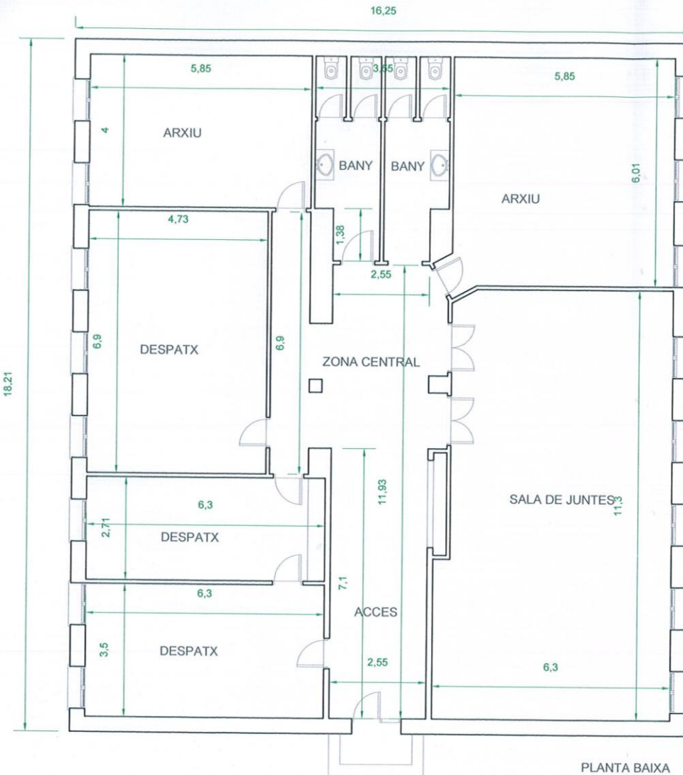
PLANTA BAIXA ESTAT ACTUAL DISTRIBUCIO COTES BASIQUES SUPERFICIES CONSTRUÏDA 295,91 mts.2
